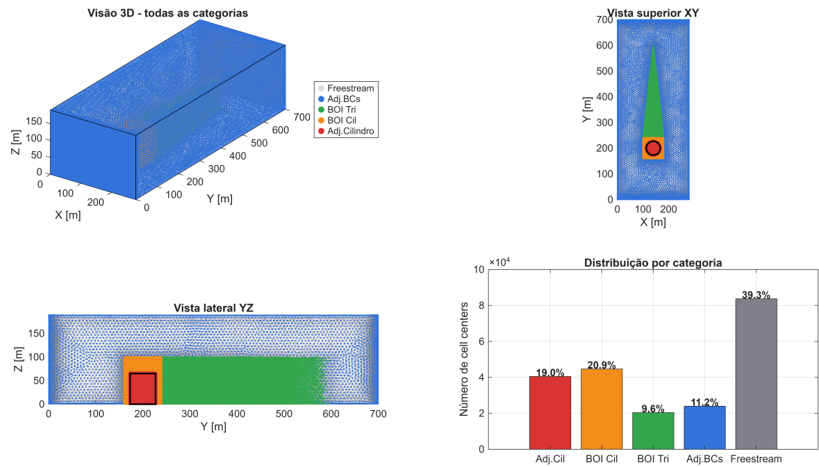
FIGURA 4: Visão Global da Distribuição (n=213146 cell centers)
