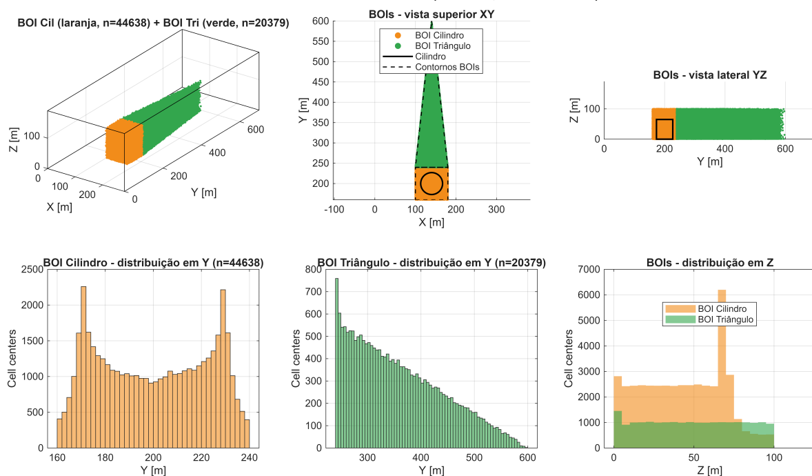
FIGURA 2: BOIs Volumétricos (n=65017, 30.5% do total)
